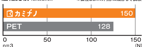
圧縮比較 (独自試験) ※直径8cmの円形に成形して試験
