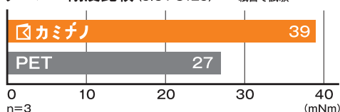
テーパー剛度比較 (JIS P8125) ※サポーターの横方向の紙目で試験
